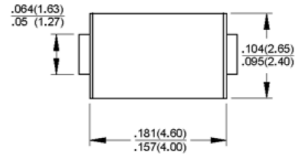
DO-214AC (SMA)
