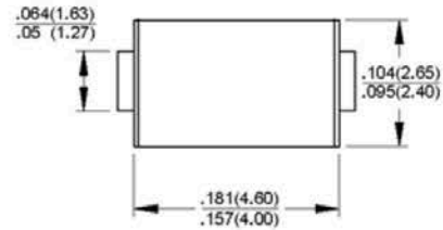
DO-214AC (SMA)
