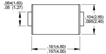
DO-214AC (SMA)
