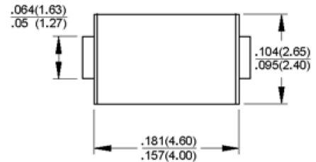
DO-214AC (SMA)
