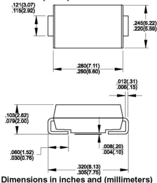
DO-214AB (SMC)
