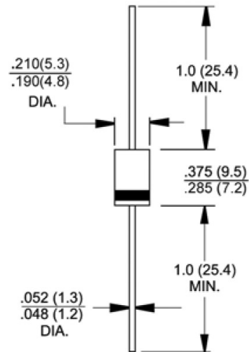
DO-201AD
