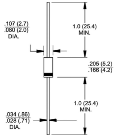
DO-204AL (DO-41)
