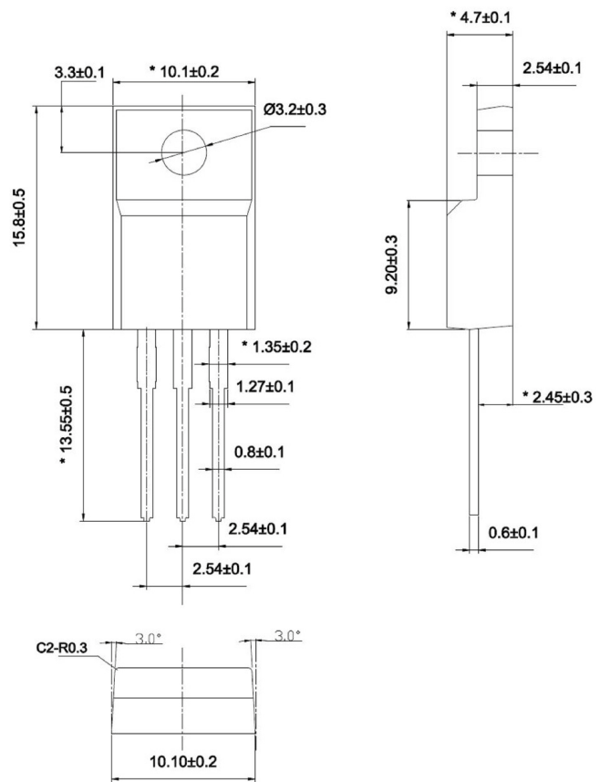
ITO-220-AB
