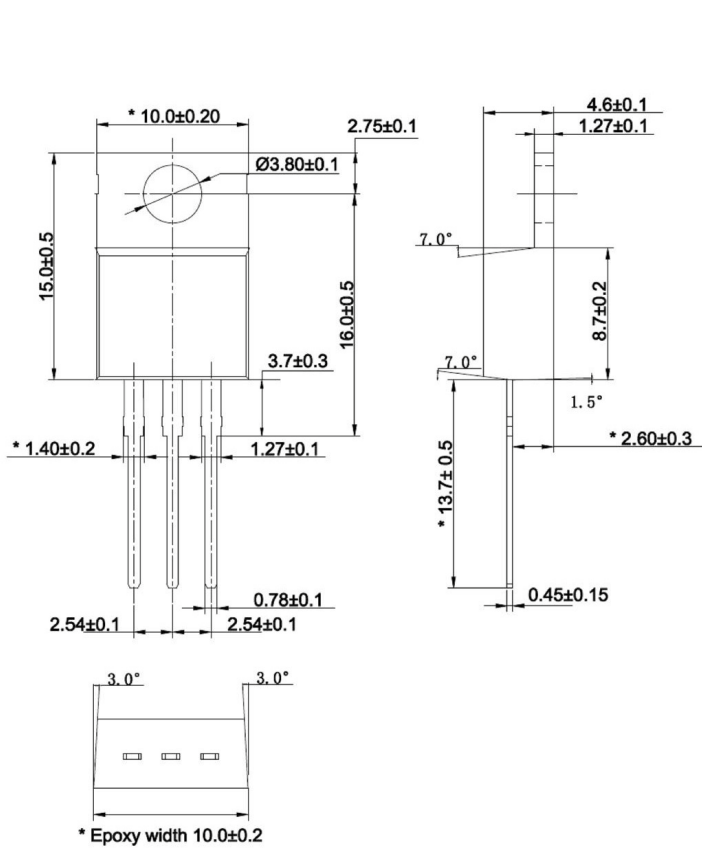
TO-220-AB
