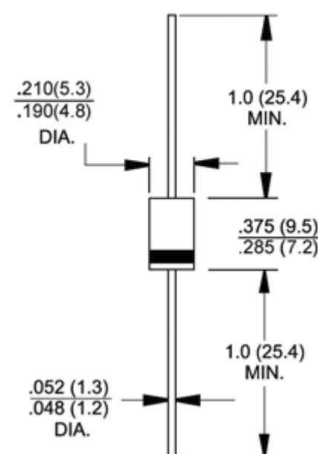
DO-201AD
