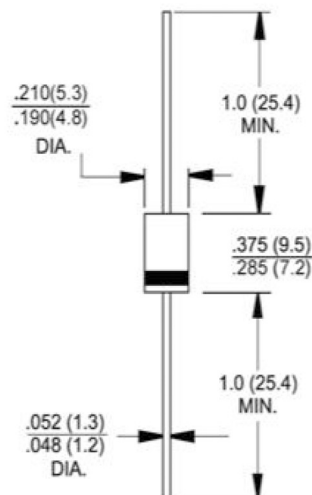
DO-201AD
