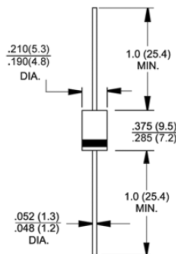
DO-201AD
