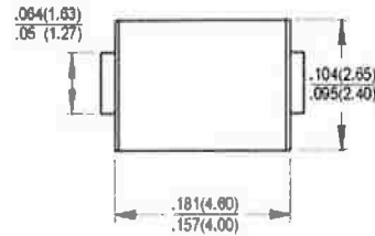
DO-214AC (SMA)
